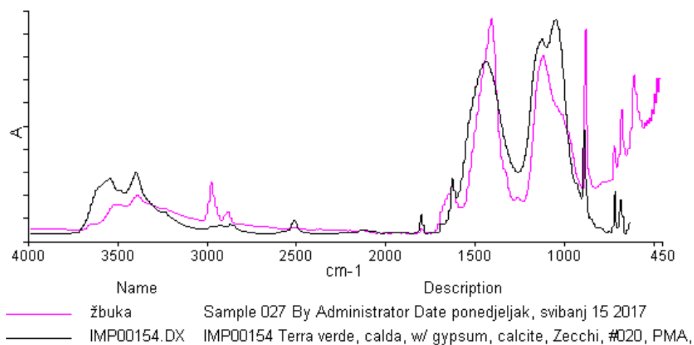
Slika 42. FTIR analiza, određivanje sastava žbuke
