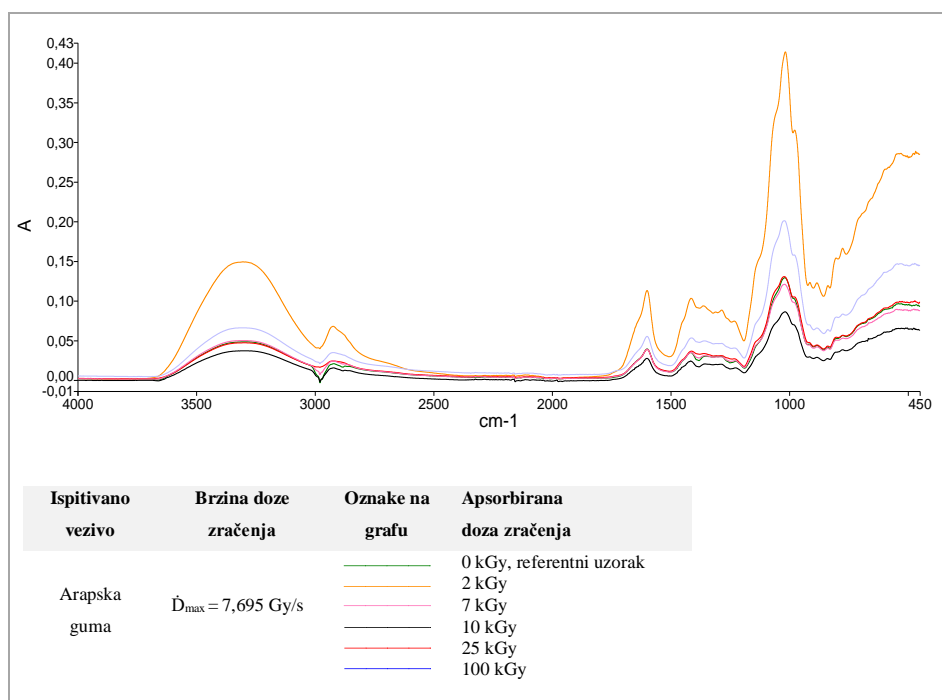
Sl. 110. rezultati analiza izvedenih FTIR uređajem na referentnom uzorku arapske gume te na uzorcima veziva arapske gume ozračenih u centru, maksimalnom brzinom zračenja ( \dot{D}_{\max} = 7,695\text{ Gy/s} )
