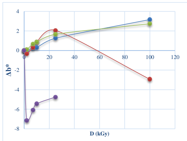
Sl. 92. Promjena kolorimetrijskog \Delta b^* parametra uzoraka (bjelanjak + olovno bijela) ozračenih odabranim dozama neposredno nakon zračenja i mjesec dana nakon zračenja neposredno nakon zračenja:
