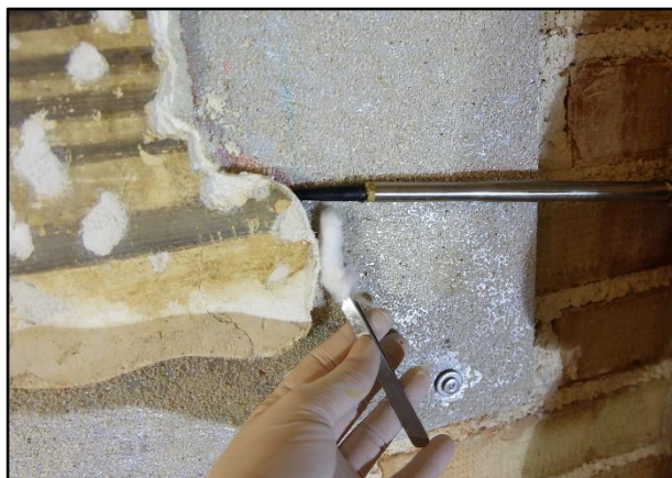
Slika 150. Injektiranje PUR pjene
