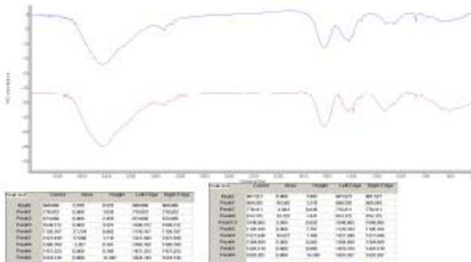
Slika 2. FT-IR spektri vodernih ekstrakata uzoraka lab. br. 20732 i 20733
