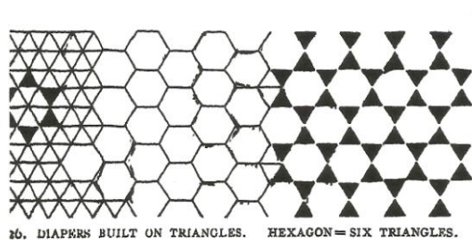
Slika 36: Konstruiranje ornamenta na osnovu trokuta; Day, 1933:19.
