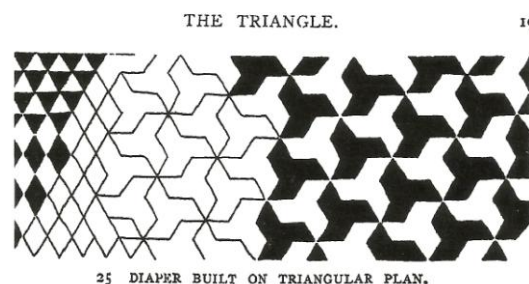
Slika 37: Konstruiranje ornamenta na osnovu trokuta; Day, 1933:19.
