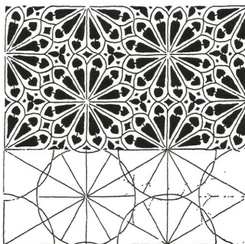
Slika 43: Primjer dekorativne forme nastale na osnovu kružnice; Day, 1933:36.
