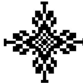
Slika 250: Forma C5 proizašla iz postupka permutiranja rotiranjem u koordinatnom sustavu s preklapanjem na uzorku J1.
