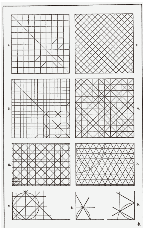
Slika 34: Pravokutna konstrukcijska mreža; Meyer (1849: 5, 10).
