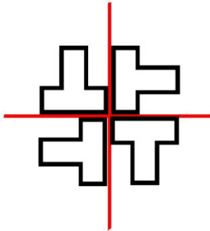
Slika 160: Permutacija rotiranjem u koordinatnom sustavu
