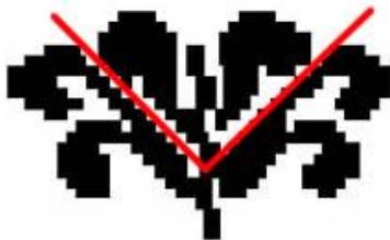
Slika 221: Dominantni pravci na uzorku D.
