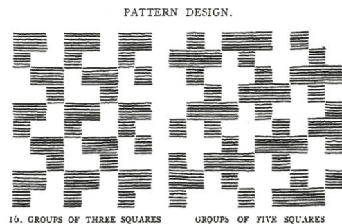
Slika 31: Primjer složenijeg pravokutnog ornamenta; Day, 1933:14
