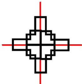
Slika 171: Prikaz permutacija rotiranjem u koordinatnom sustavu s preklapanjem.
