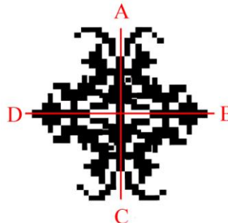
Slika 172: Permutiranje rotiranjem u koordinatnom sustavu s preklapanjem na uzorku G2.
