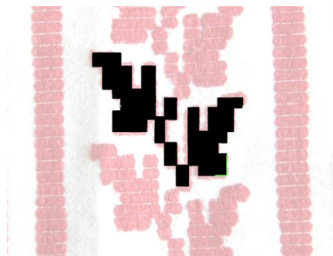
Slika 92: Pozicija ornamentalnog uzorka stiliziranog lista vinove loze.
