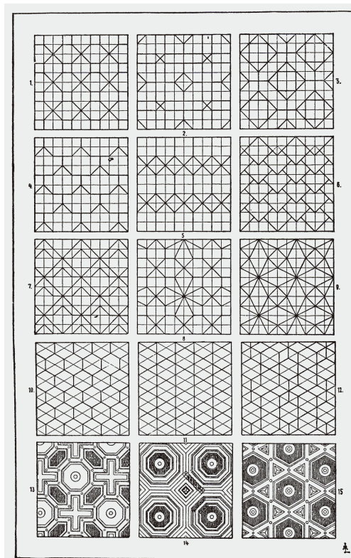
Slika 34: Pravokutna konstrukcijska mreža; Meyer (1849: 5, 10).
