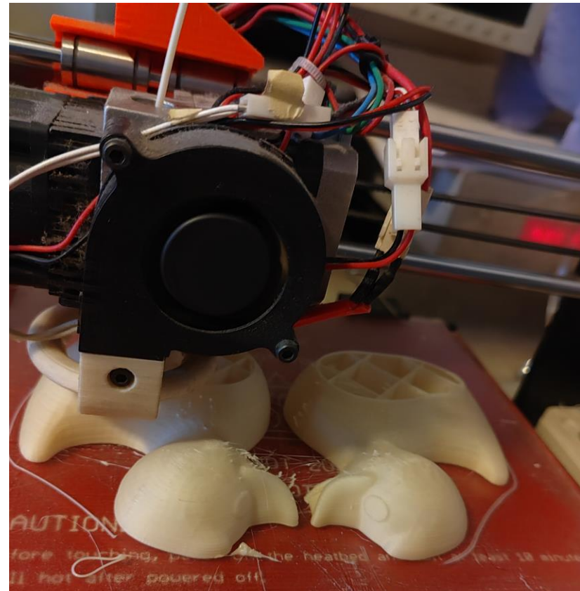
Slika 12 - Printanje osnovnog modela na 3D printeru
