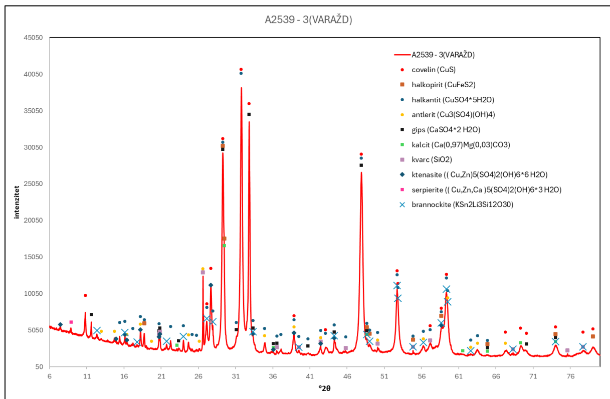
Slika 101. XRD spektar korozivjske kore kovanice A3
