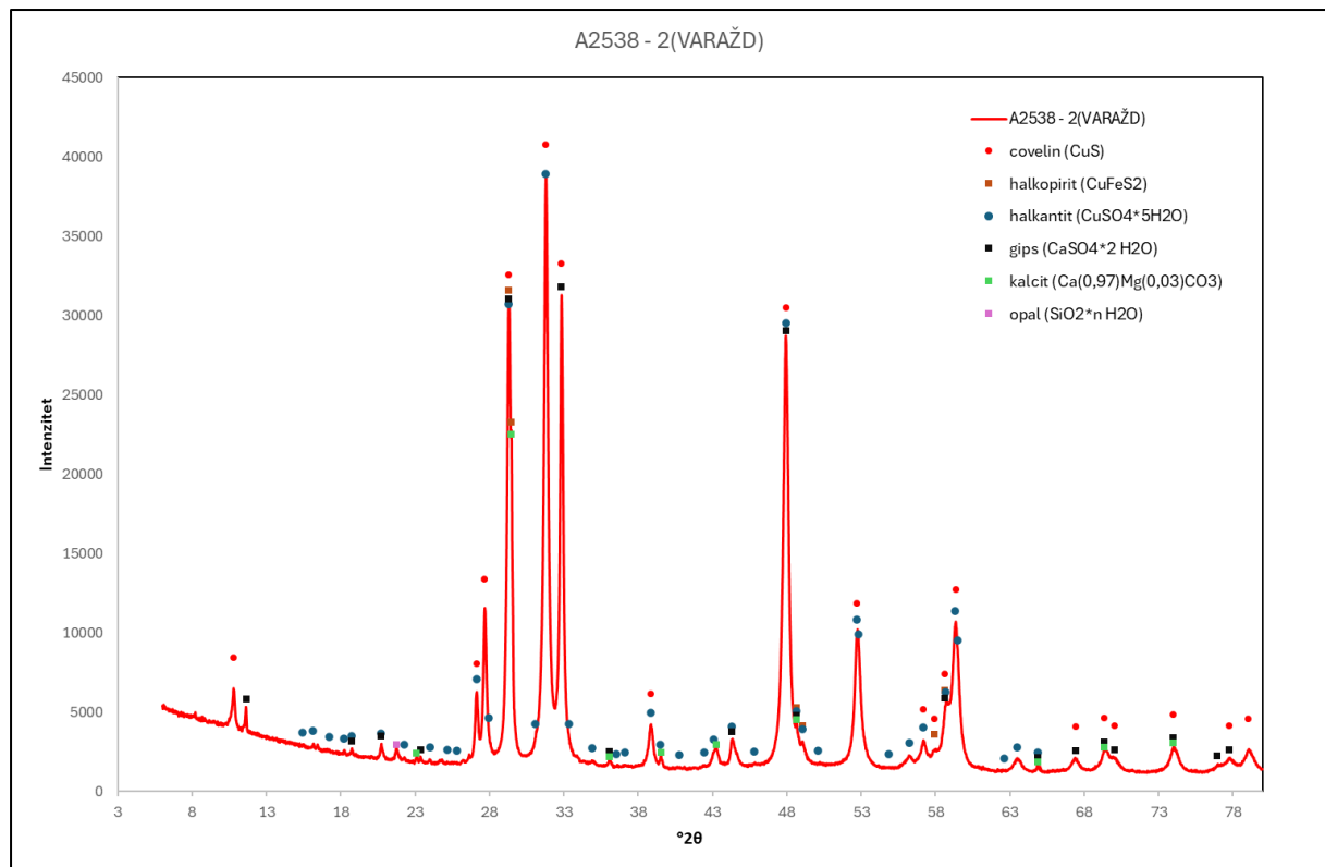
Slika 100. XRD spektar korozivjske kore kovanice A2
