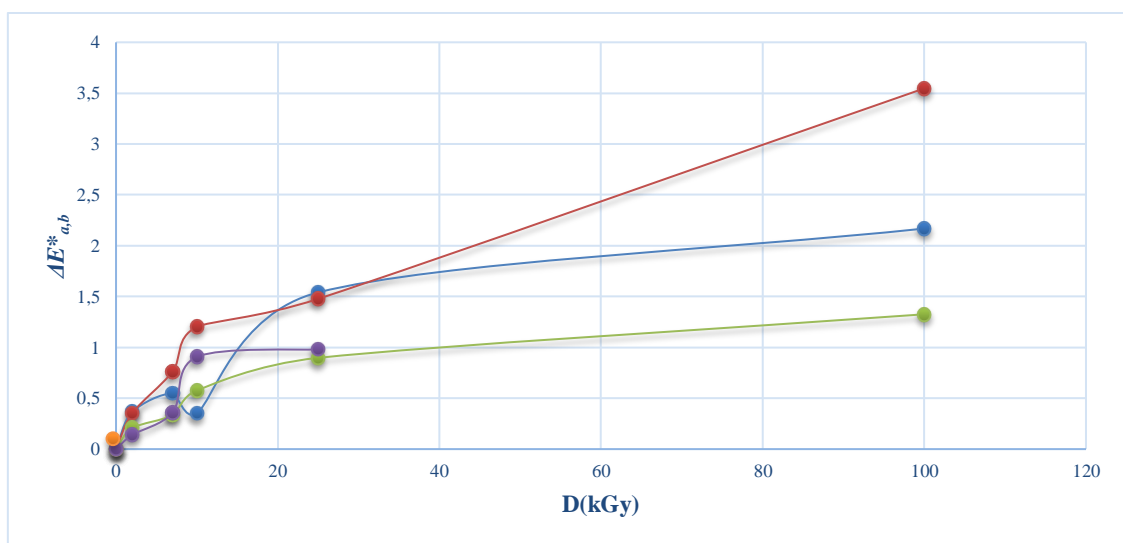
Sl. 109. Promjena kolorimetrijskog \Delta E_{a,b}^* parametra uzoraka (tutkalo + olovno bijela) ozračenih odabranim dozama neposredno nakon zračenja i mjesec dana nakon zračenja neposredno nakon zračenja:
