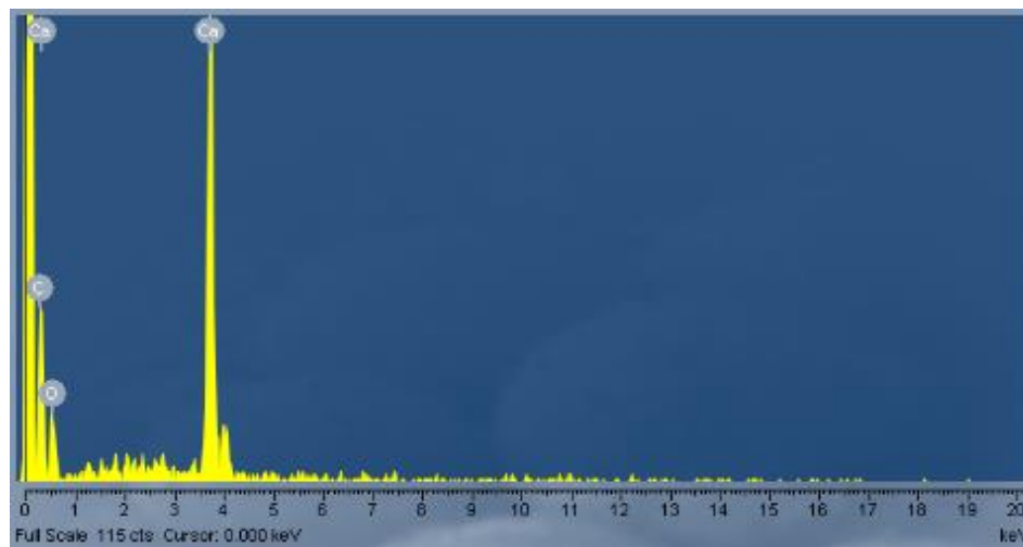
Slika 2. Fragment1/uzorak1/VZ1/sljubnica, rezultat veziva dobiven pomoću (skenirajućeg) elektronskog mikroskopa (SEM-a)
