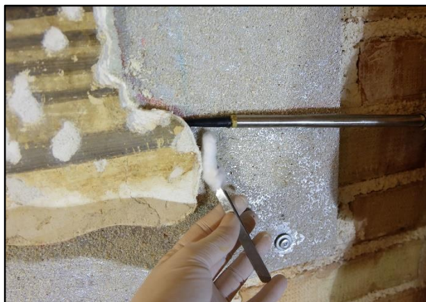
Slika 150. Injektiranje PUR pjene
