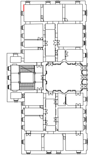
Tlocrt kata
