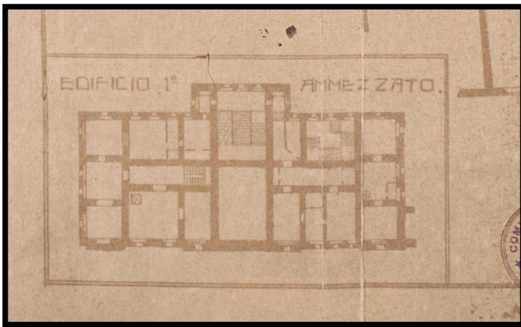
Slika 7 Palača Šećerane, tlocrt s ucrtanim stubištem
